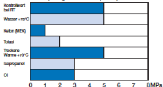
Alterungsbeständigkeit von PP-Verklebungen
