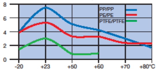
Festigkeitsentwicklungen von WEICON Easy-Mix PE-PP an Zugscherproben nach DIN 53283
