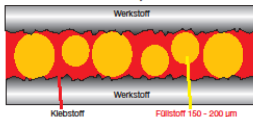
Graphische Darstellung einer Klebefuge mit WEICON Easy-Mix PE-PP
