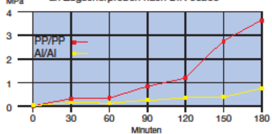
Alterungsbeständigkeit von PE-Verklebungen
